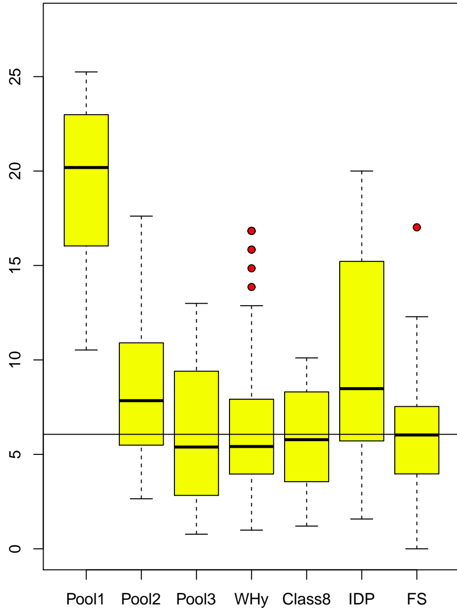
pctE vs group
