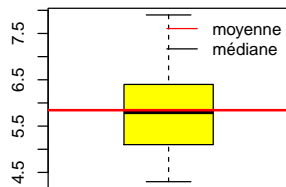
Boite à moustaches pour sepal.len (cm)
