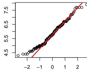
Droite de Henry pour sepal.len (cm)
